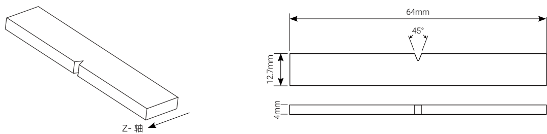
图3. 抗撕裂测试样条
