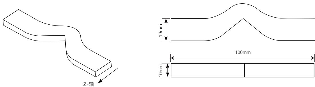
图3. 抗撕裂测试样条
